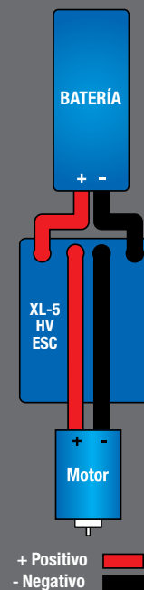
Diagrama de cableado del XL-5 HV
